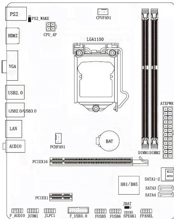
1-3 主板布局图
